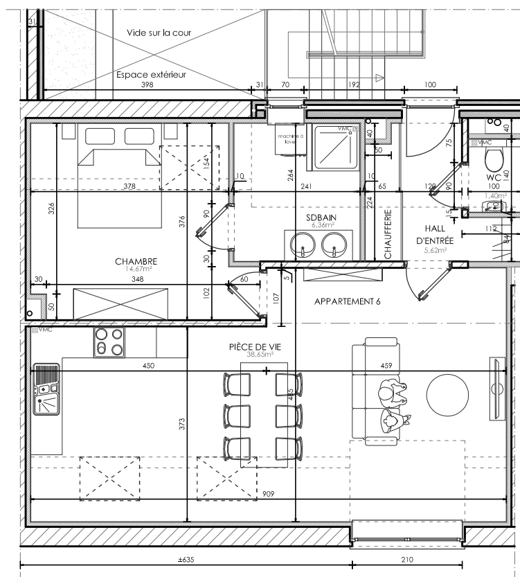
APPARTEMENT 6
